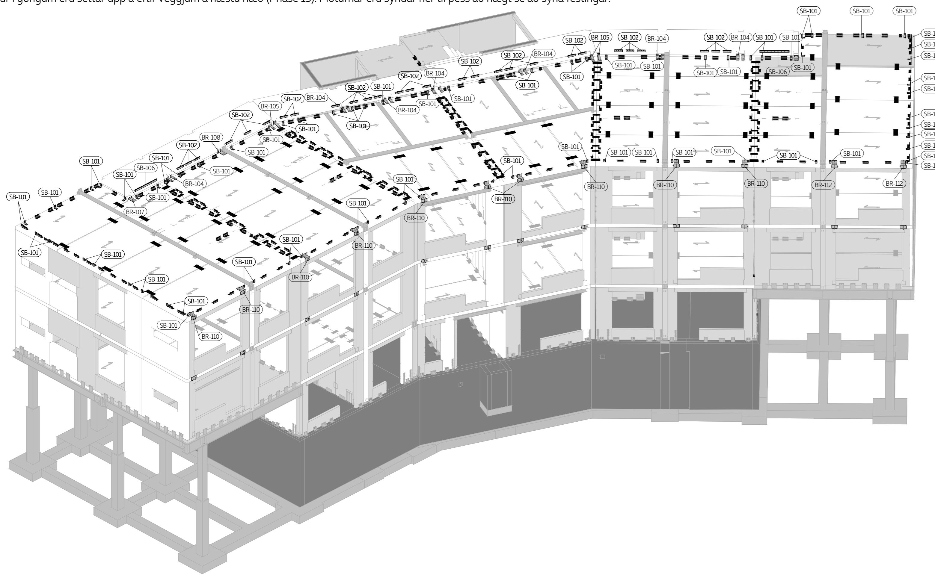
13 - Þrívídd - 4. hæð - Festingar
