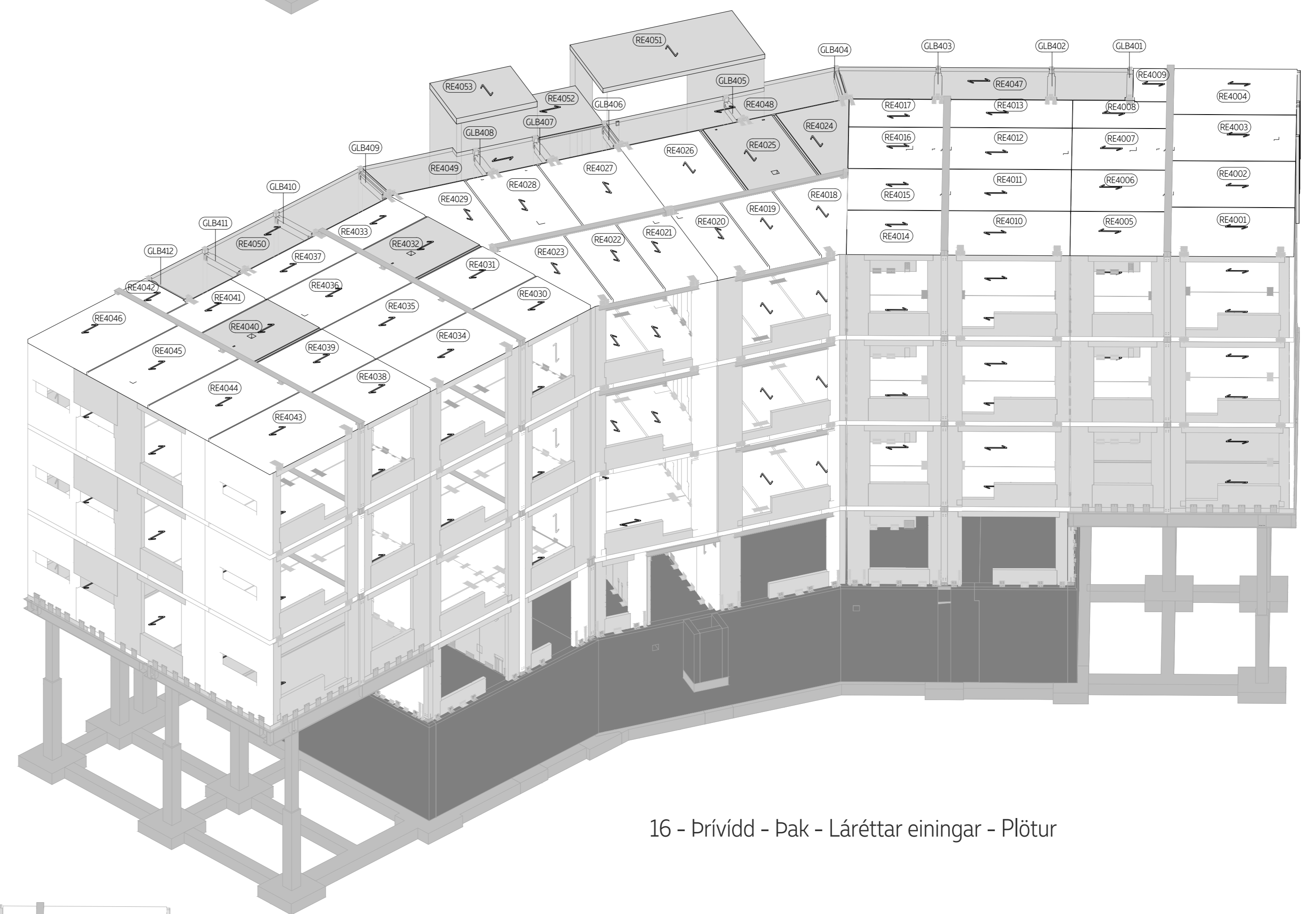
14 - Þrívídd - 4. hæð - Lóðréttar einingar
