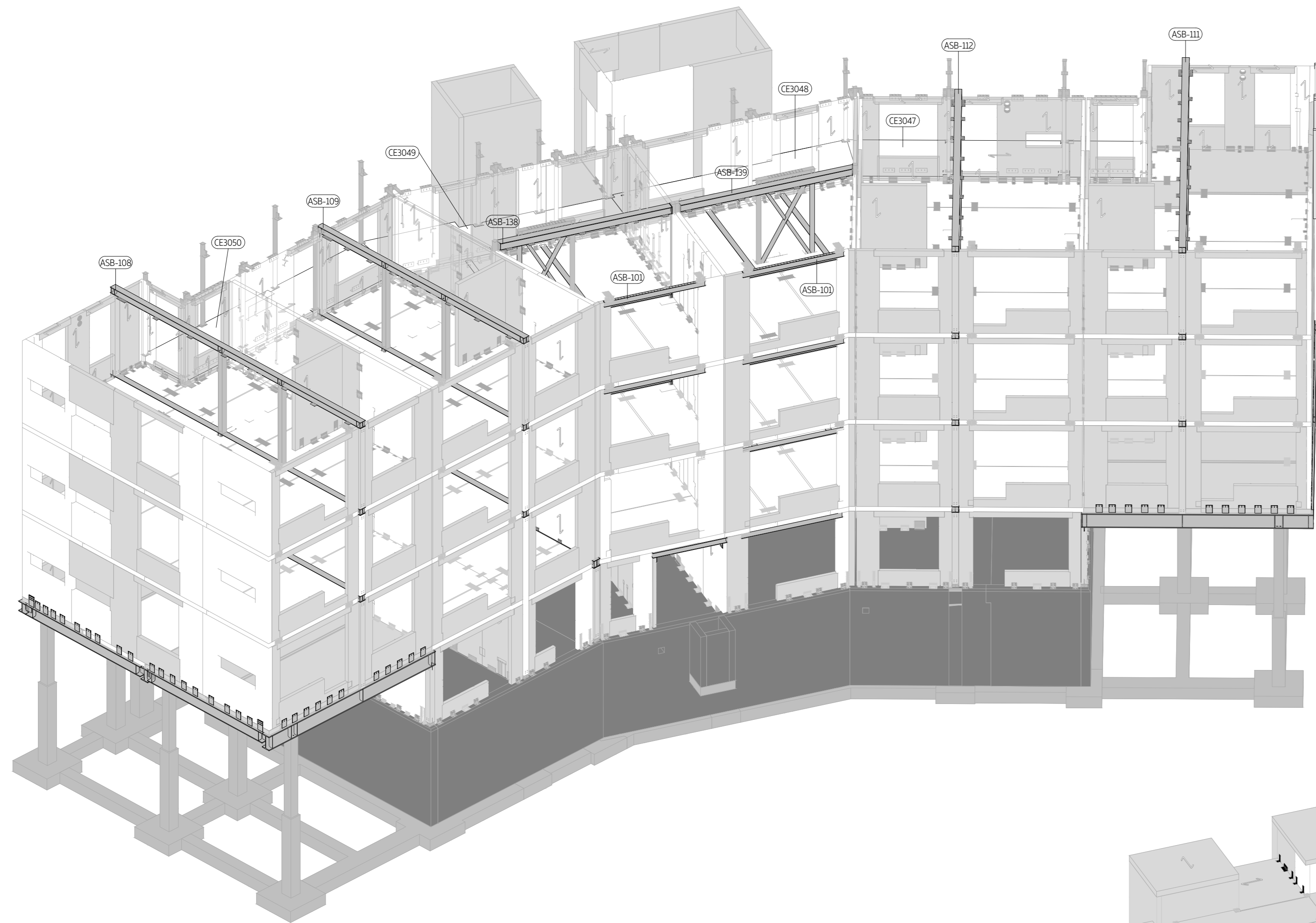
15 - Þrívídd - Þak - Láréttar einingar - Bitar og plötur á göngum
